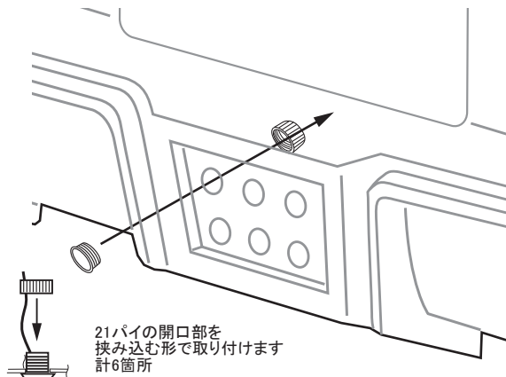
■LED 取り付け説明図
