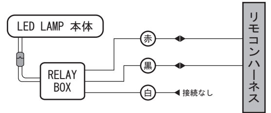
図1 = 配線図 =
