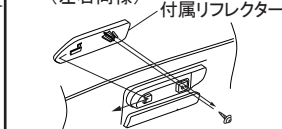
図3 リフレクター部リアスカート裏面図(左右同様)
