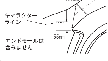
図2 フロントオーバーフェンダー 参考位置図
