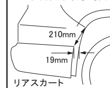
図3 リフレクター部リアスカート裏面図(左右同様)
